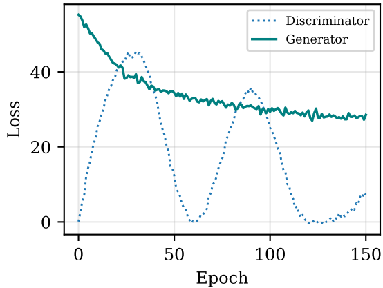
EuroSAT
